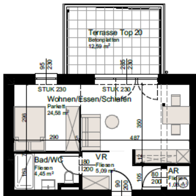
▲ TOP 20 35,20 m 2
